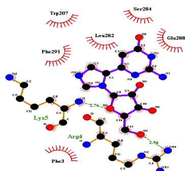
compound a: using ligplot
